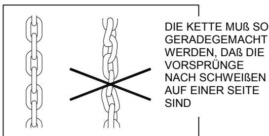
Abb. 1 Verdrehung der Kette
