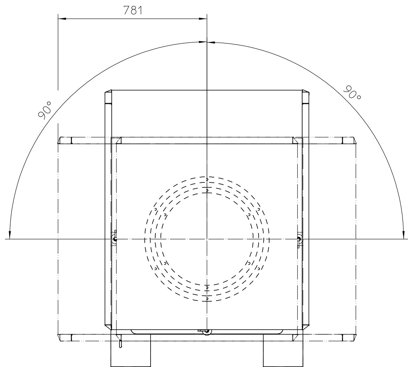
Draufsicht Maßstab 1:12
