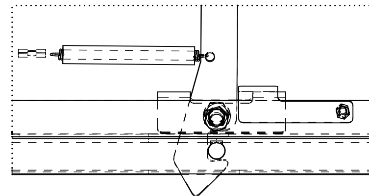
Detail1 Maßstab 1:4
