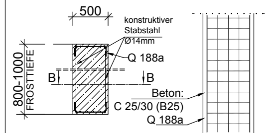
Schnitt "A"-"A"
