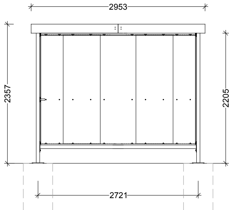
Vorderansicht
