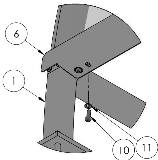
DETAIL L 1 : 5
