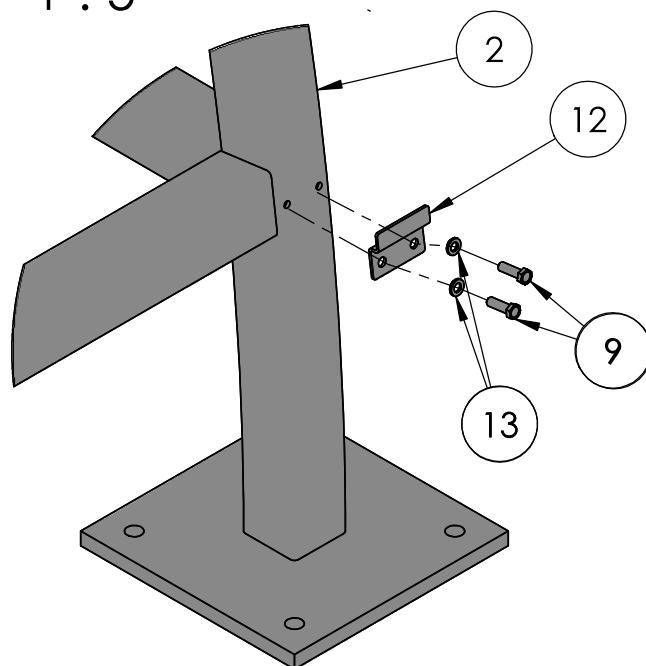
DETAIL F 1 : 5
