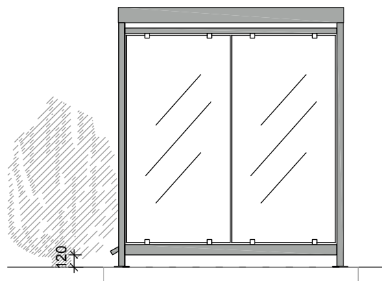
Seitenansicht
