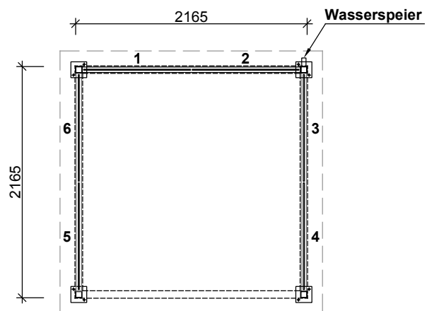
Grundriss
