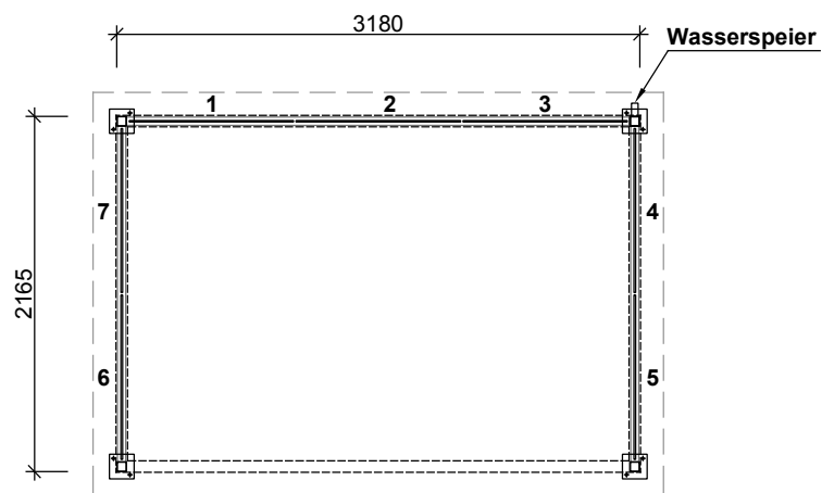
Grundriss
