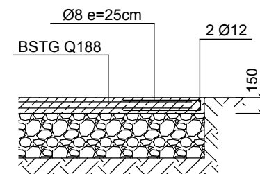
(Fertig-) Bodenplatte
