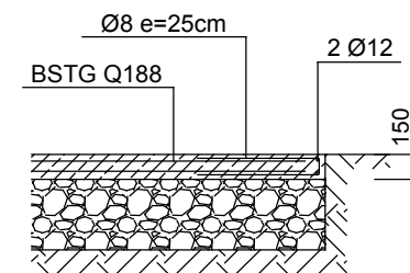
(Fertig-) Bodenplatte
