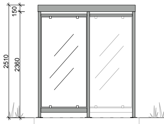
Vorderansicht
