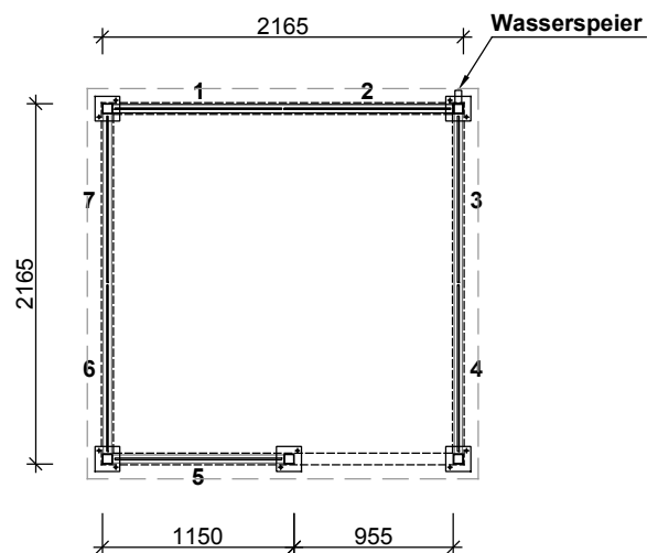
Grundriss
