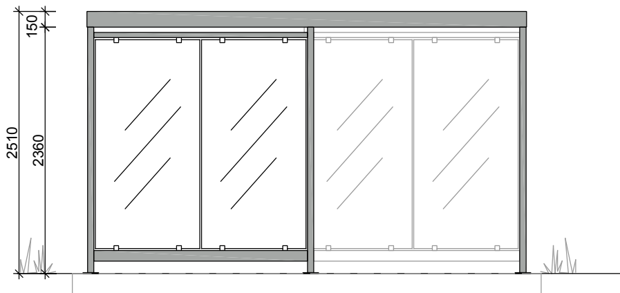
Vorderansicht
