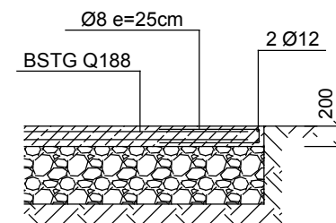
(Fertig-) Bodenplatte
