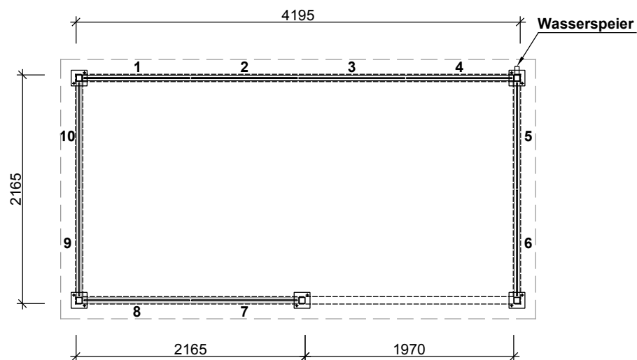
Grundriss
