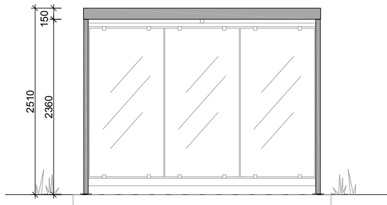
Vorderansicht
