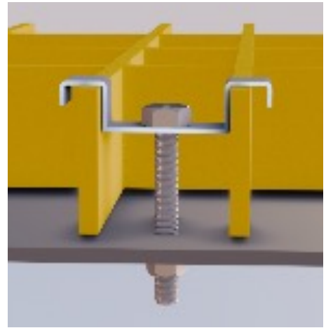
M-Klemme
