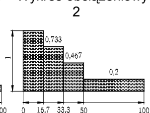
Wykres obciążeniowy
