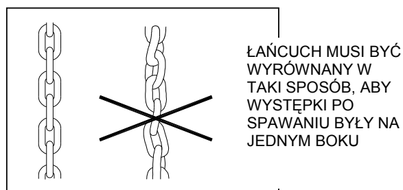
Obr. 6.2a Skręcenie łańcucha
