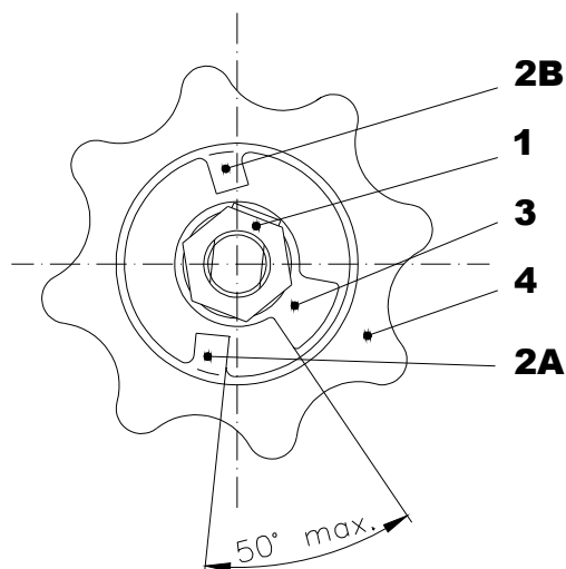
Rys. 11.4 – Regulacja hamulca
