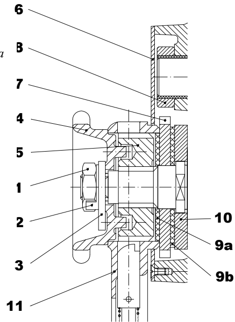
Obr. 11.3 - Montáž brzdy
